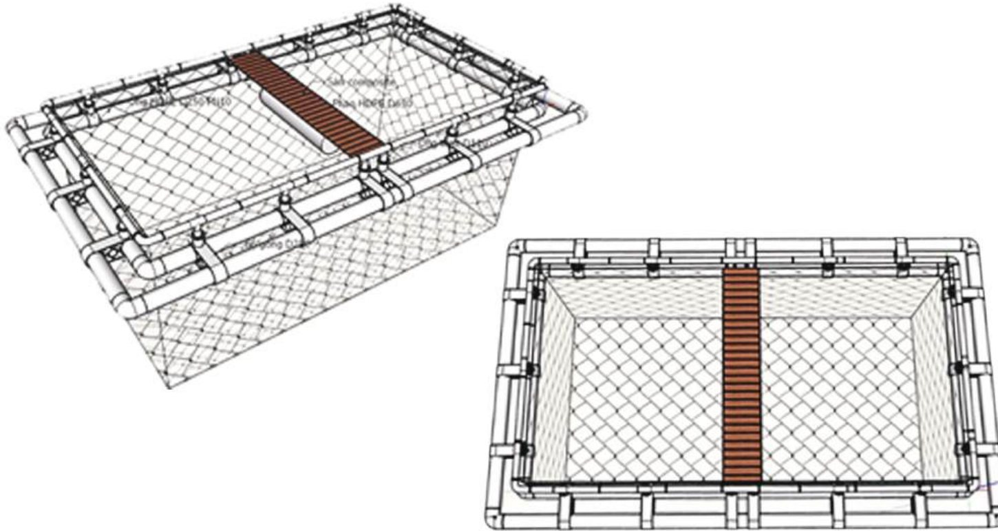
Bản vẽ kỹ thuật lồng chữ nhật HDPE của STP
