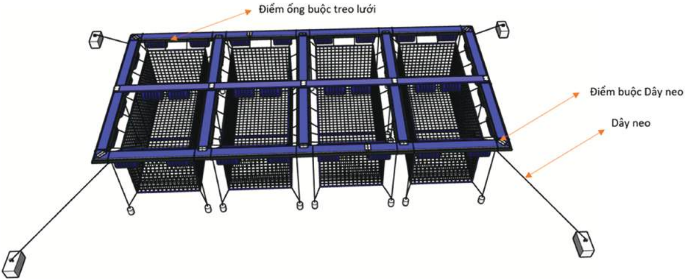
THÔNG SỐ KỸ THUẬT CỦA CỤM 1 Ô LỒNG PHAO HẠ TẦNG 4X8M
