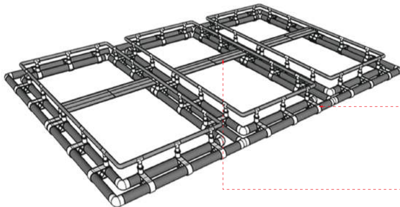
LỒNG CHỮ NHẬT HDPE
